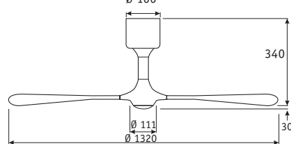
HELICO PADDEL
